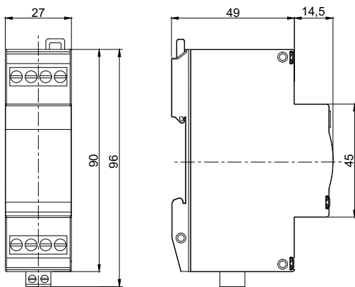
Габаритные размеры
